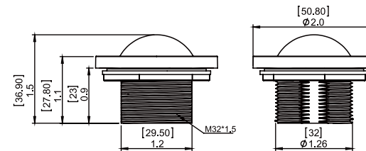
(sensor antenna)
