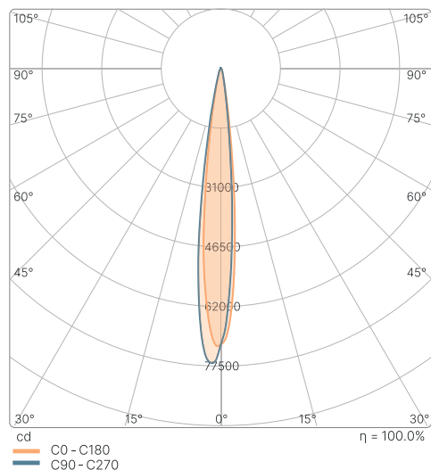
8" / 58W / 3000K / NARROW 15°
