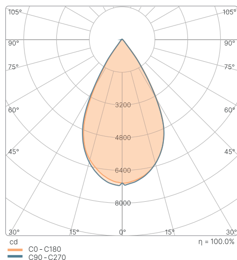
8" / 58W / 3000K / FLOOD 60°
