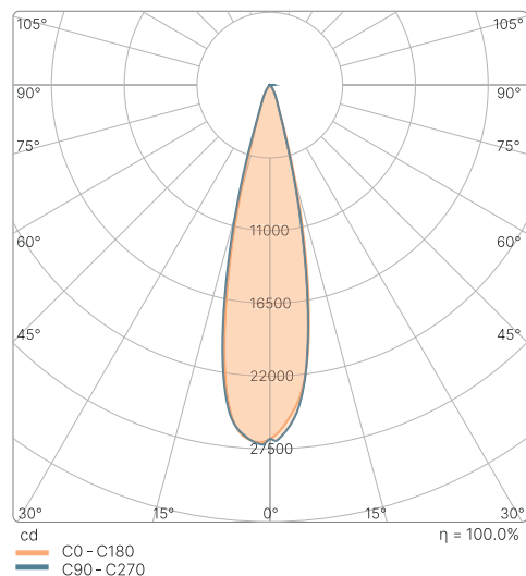
8" / 58W / 3000K / MEDIUM 24°
