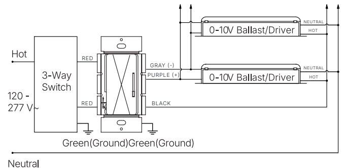
3-WAY WIRING
